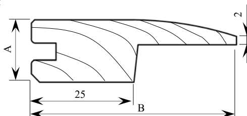
Рисунок 4: Ковровый порожек
