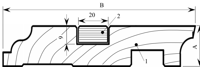
Рисунок 1: Плинтус №11 - поперечный профиль 1- массив березы сращенный по длине 2- декоративная вставка из фанеры
