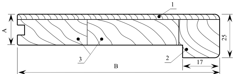
Рисунок 1: Ступенька
