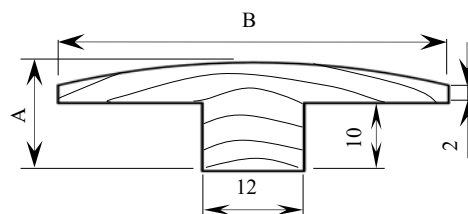
Рисунок 2: Т-молдинг
