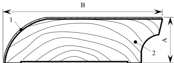
Рисунок 1: Плинтус №7
