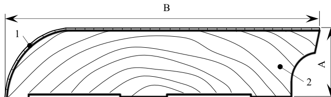
Рисунок 2: Плинтус №8
