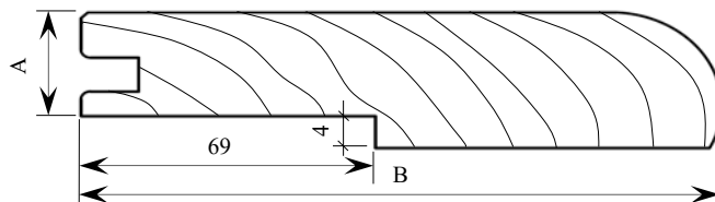
Рисунок 2: Ступенька (О-3К)
