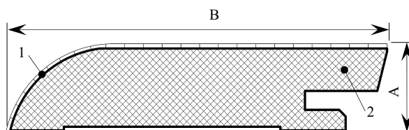
Рисунок 3: Плинтус №10
