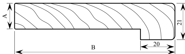
Рисунок 1: Ступенька (О-2К)
