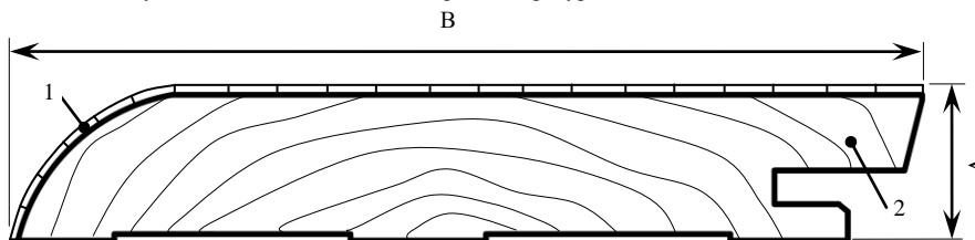
Рисунок 1: поперечный профиль Плинтуса №9 (Пл-9Шп)
