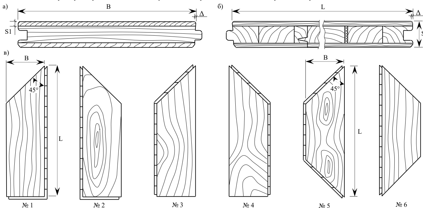
Рисунок 1: а) поперечный профиль элементов с замком типа T&G (паз-гребень); б) продольный профиль элементов с замком типа T&G (паз-гребень); в) внешний вид элементов рисунка «Кофейное зерно».
