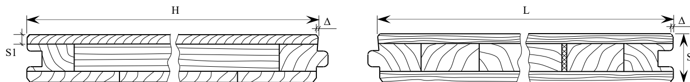
Рисунок 1: поперечный и продольный профиль модульного паркета с замком типа Т&G (паз-гребень)
